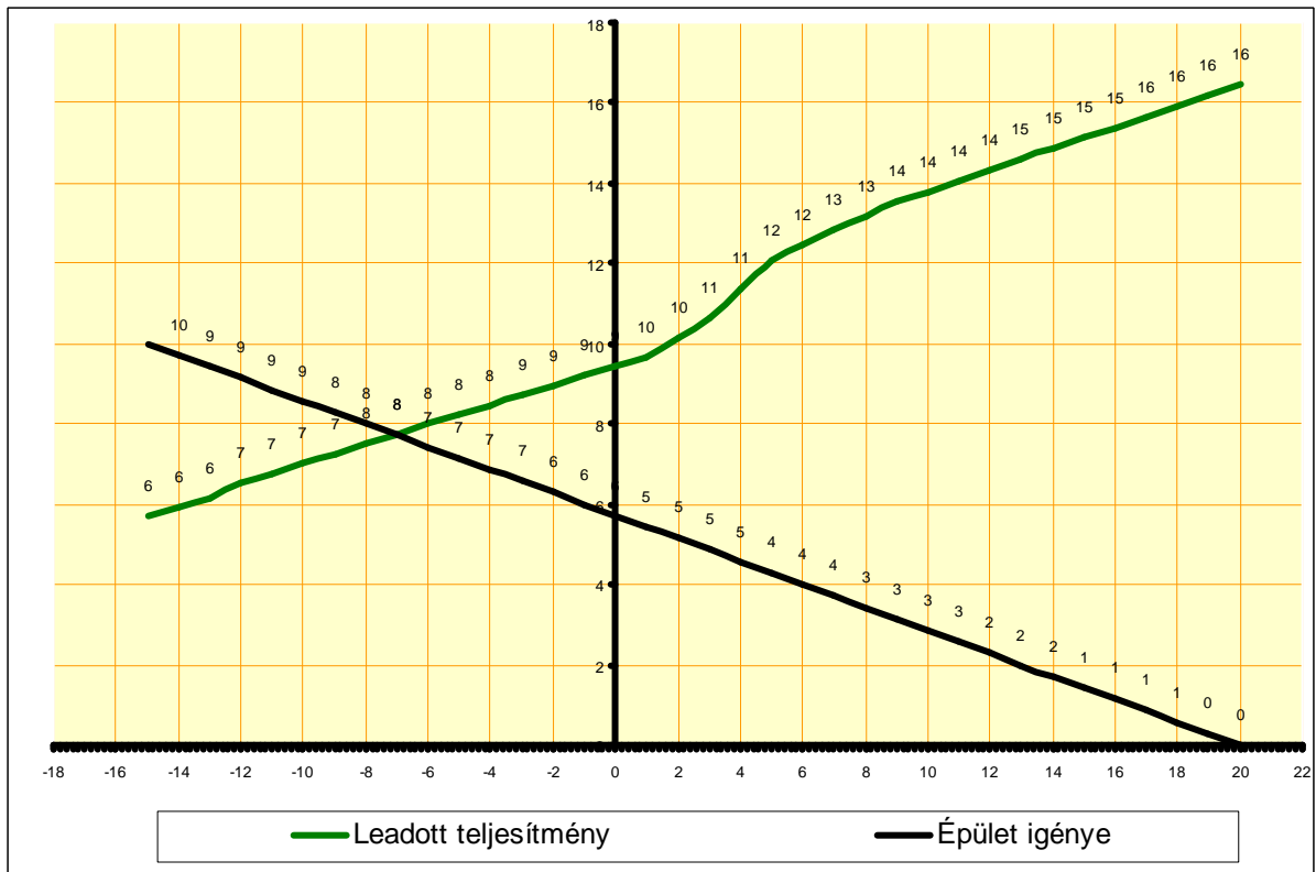
A vízszintes tengelyen a külső hőmérséklet (°C), a függőlegesen a teljesítményeket ábrázoltuk (kW).
